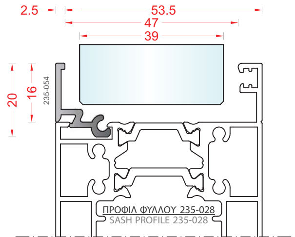
235-054 ΠΗΧΑΚΙ ΦΥΛΛΟΥ SASH GLAZING BEAD
