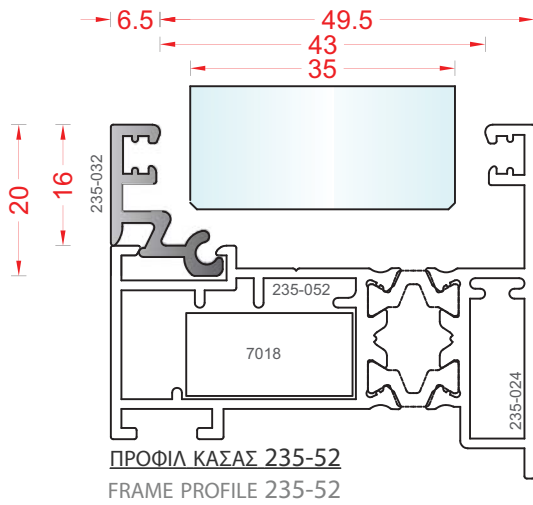
235-032 ΠΗΧΑΚΙ ΚΑΣΑΣ FRAME GLAZING BEAD
