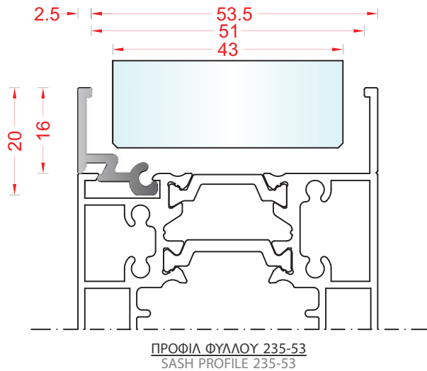
235-054 ΠΗΧΑΚΙ ΦΥΛΛΟΥ SASH GLAZING BEAD
