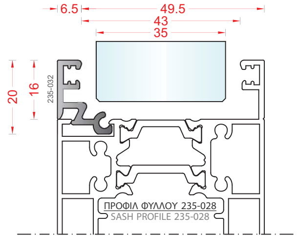
235-032 ΠΗΧΑΚΙ ΦΥΛΛΟΥ SASH GLAZING BEAD
