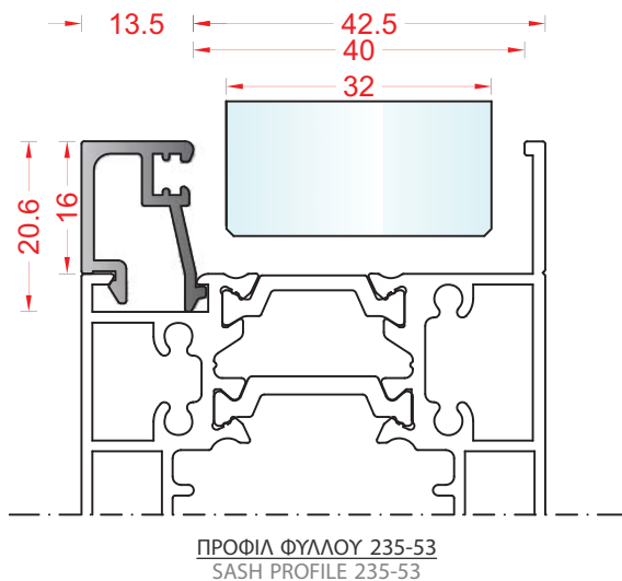
235-056 ΠΗΧΑΚΙ ΦΥΛΛΟΥ SASH GLAZING BEAD
